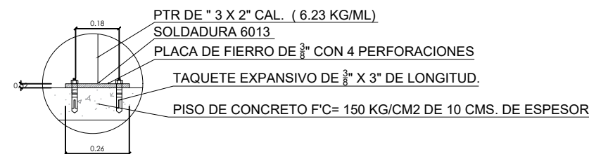
DET-07 PLACA DE POSTE ESC. 1:10
