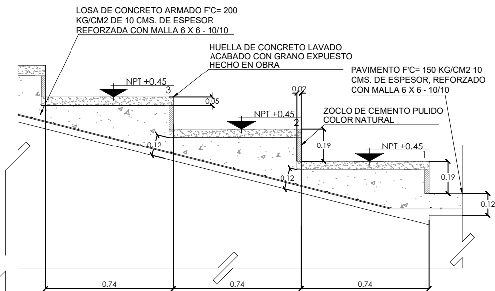
DET-04 DETALLE DE ESCALONES ESC. 1:10
