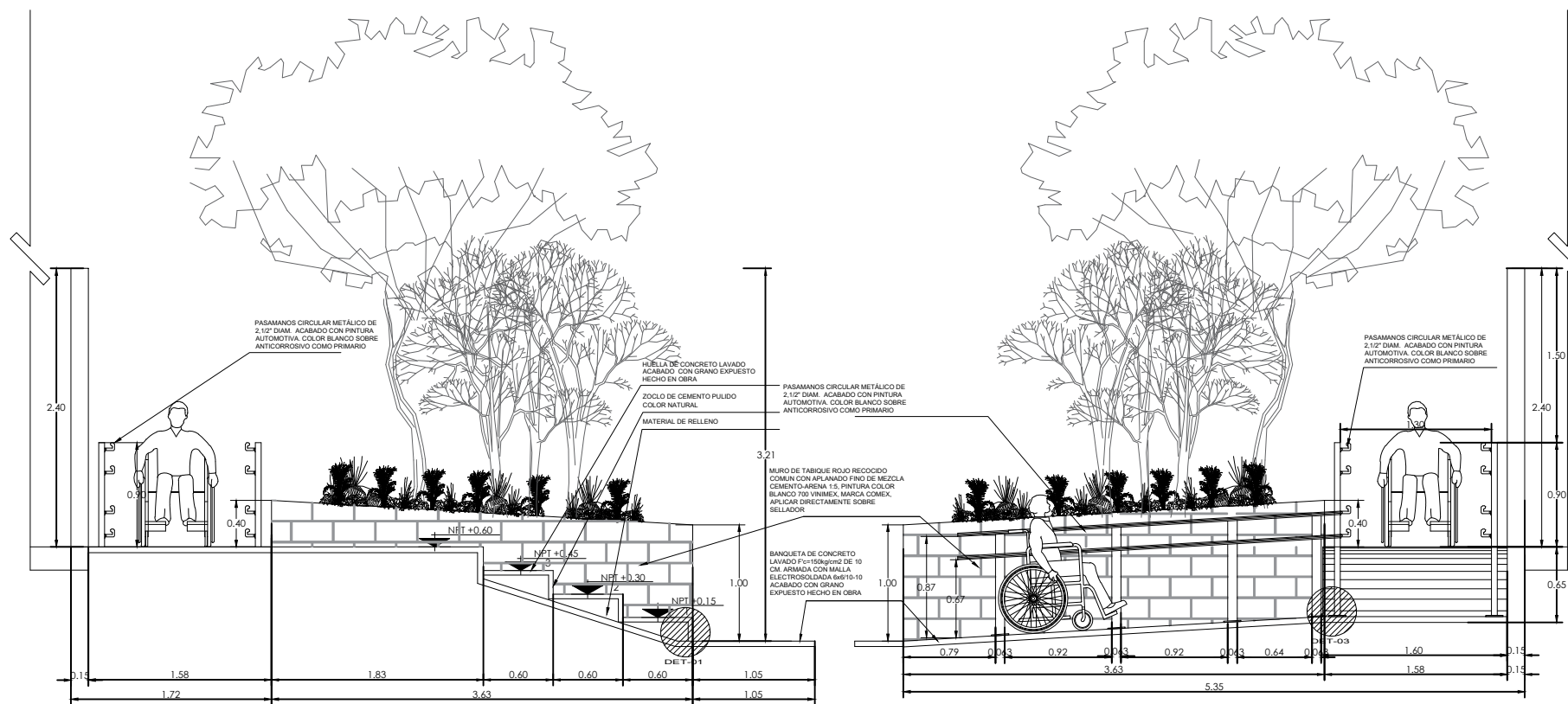
CORTE B-B' ESC. 1:25
