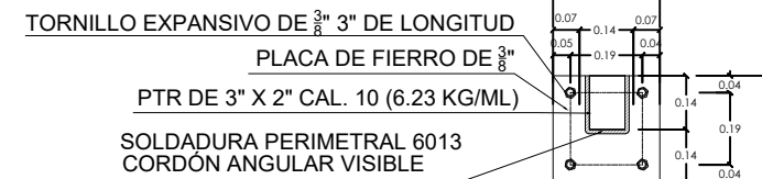
DET-03 PLACA DE ANCLAJE DE BARANDAL A PISO ESC. 1:10
