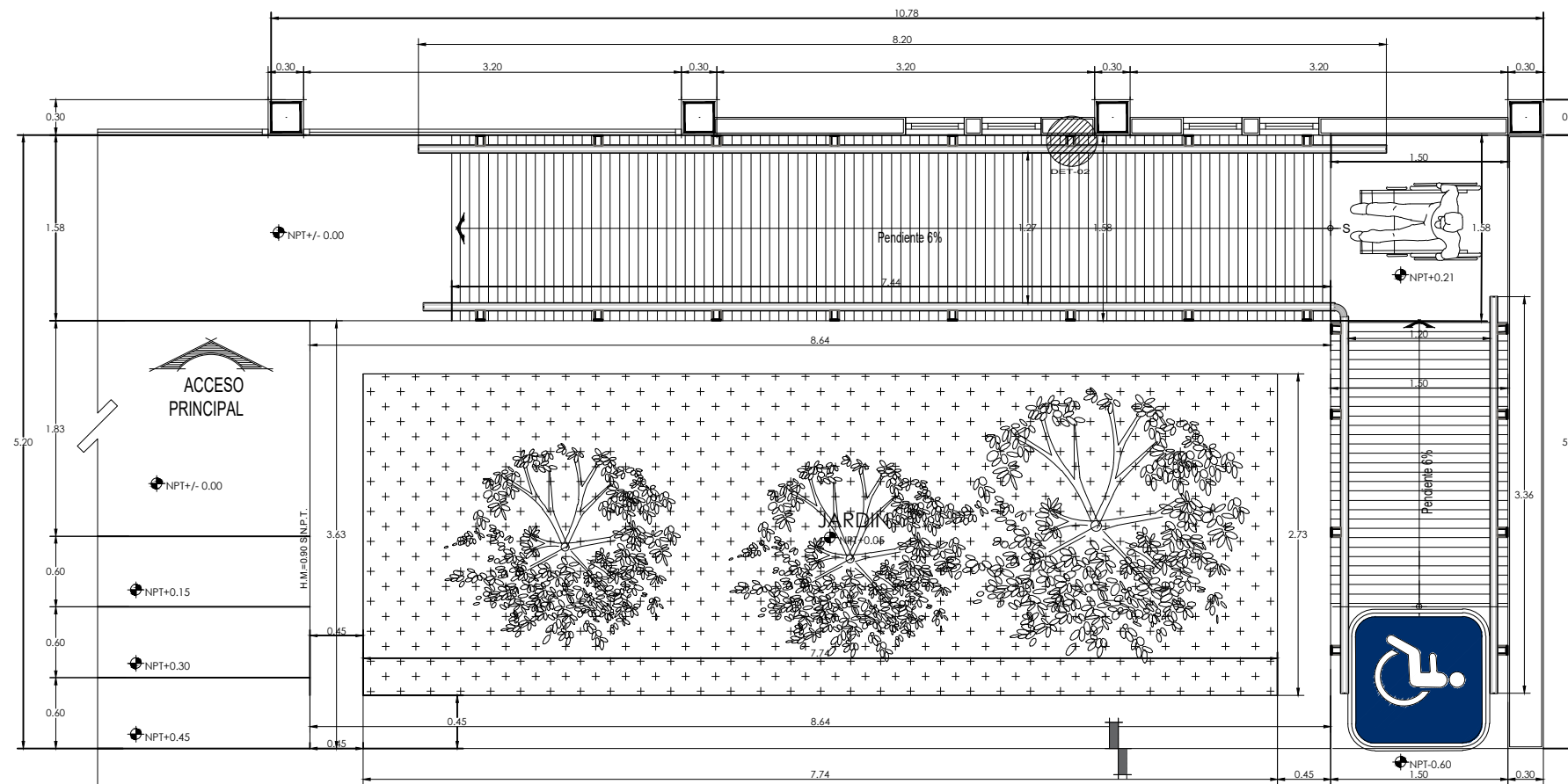
PLANTA ESC. 1:25
