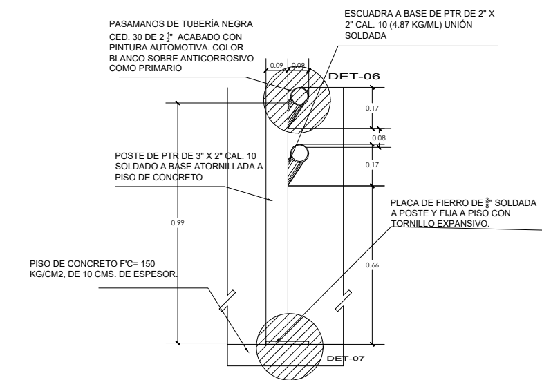
DETALLE DE POSTE DE BARANDAL ESC. 1:10
