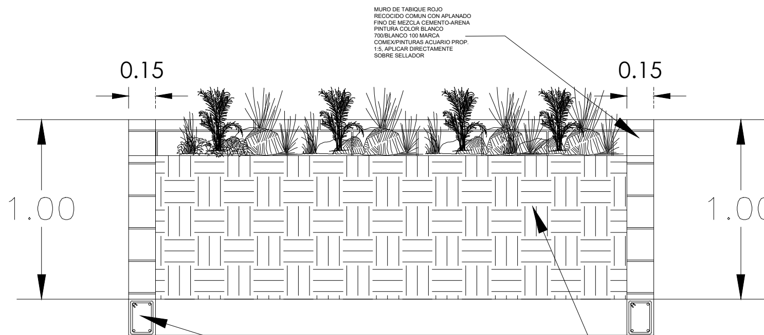
DETALLE DE JARDINERA COTAS EN MTS. ESC. 1:10
