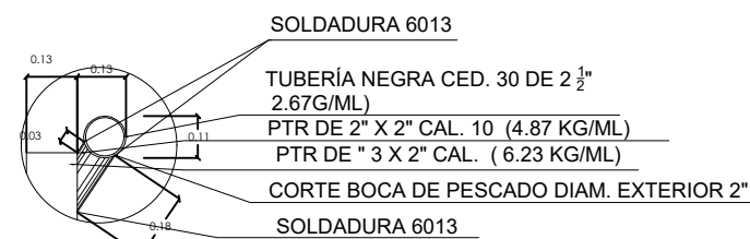
DET-06 UNIÓN DE PASAMANOS ESC. 1:10
