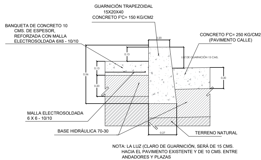
DET-01 GUARNICIÓN Y BANQUETA ESC. 1:10
