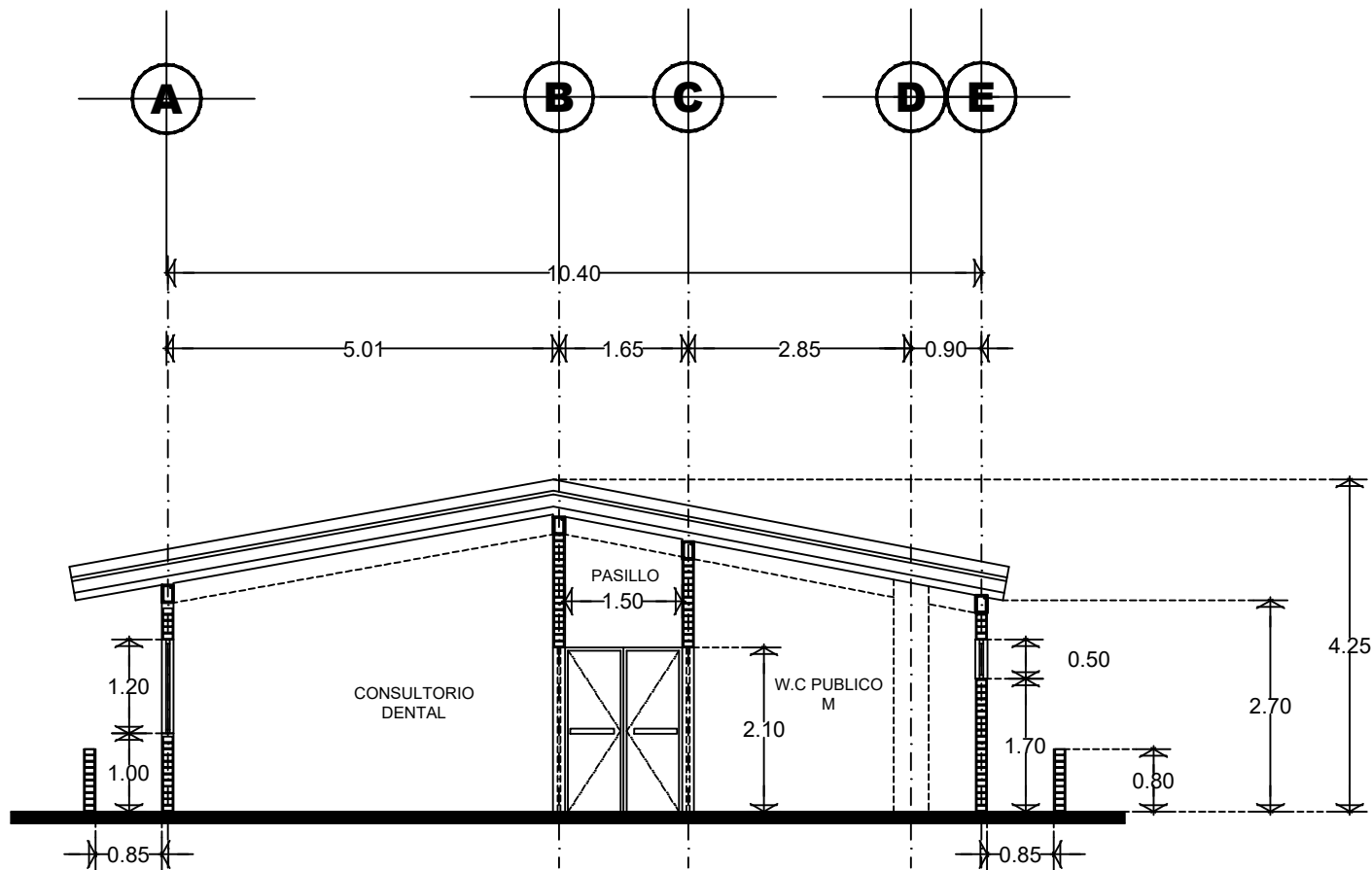
CORTE TRANSVERSAL A-A'
