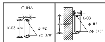
DETALLE DE UBICACIÓN DE CUÑA CON CELOTEX, EN CABEZA DE MURO QUE VAN ADOSADAS A COLUMNAS.
