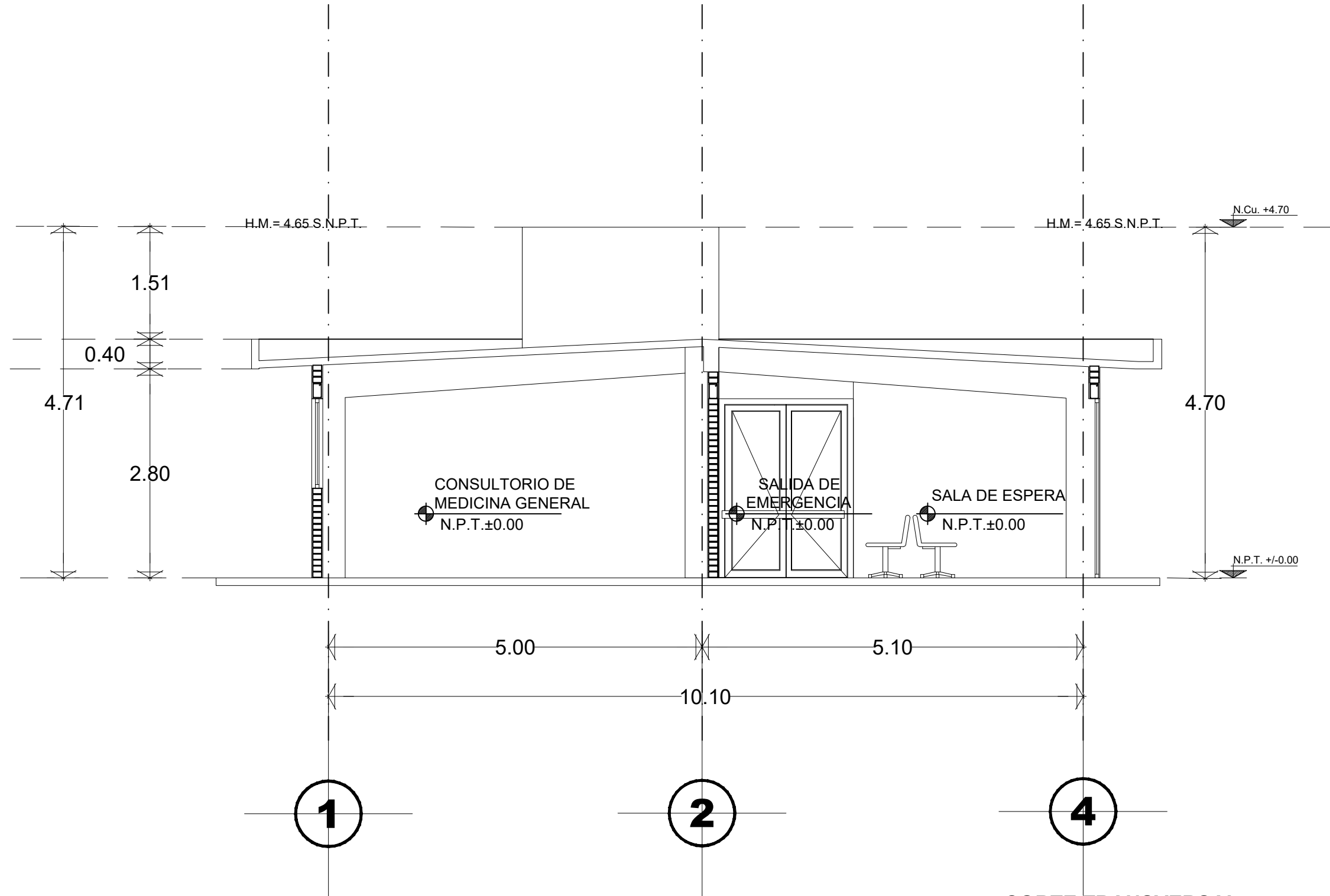
CORTE TRANSVERSAL
