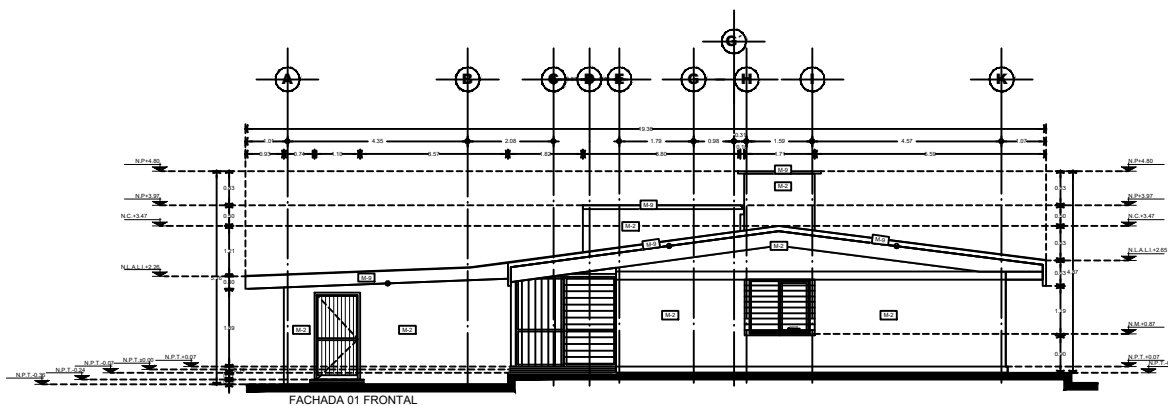
FACHADA 01 FRONTAL
