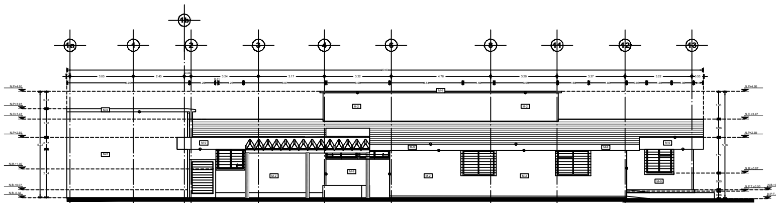
FACHADA 02 LATERAL
