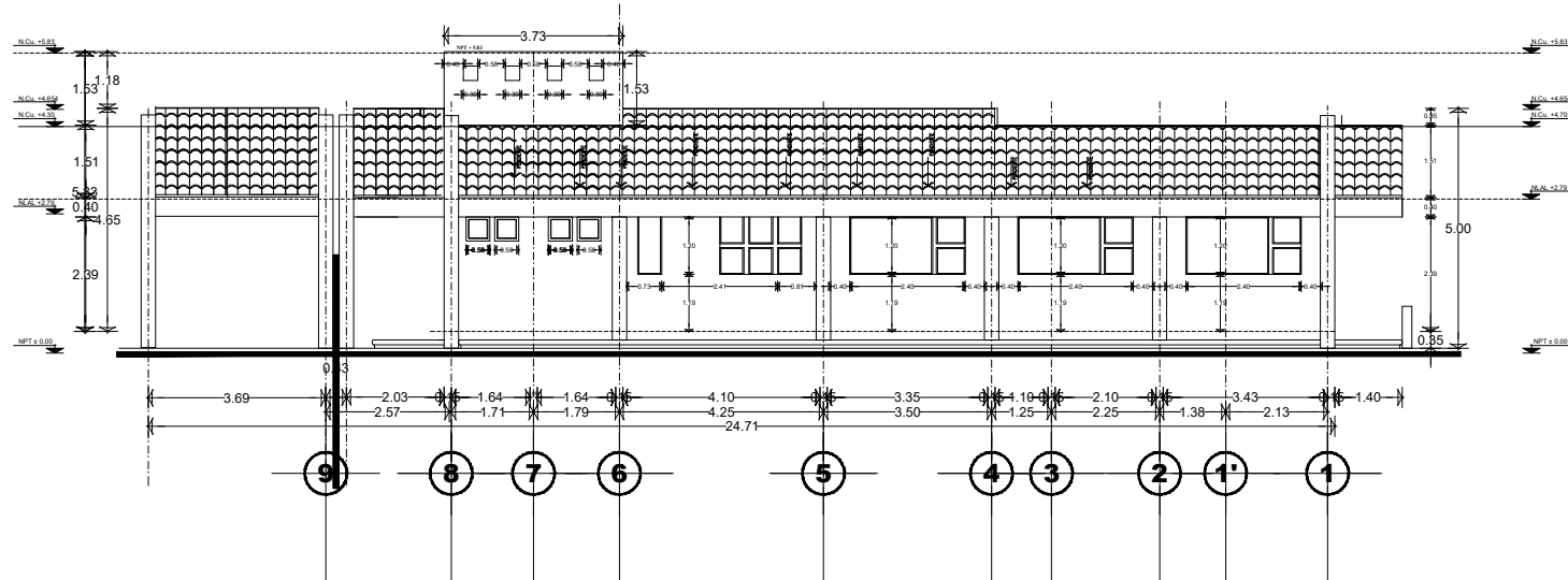
FACHADA SECUNDARIA
