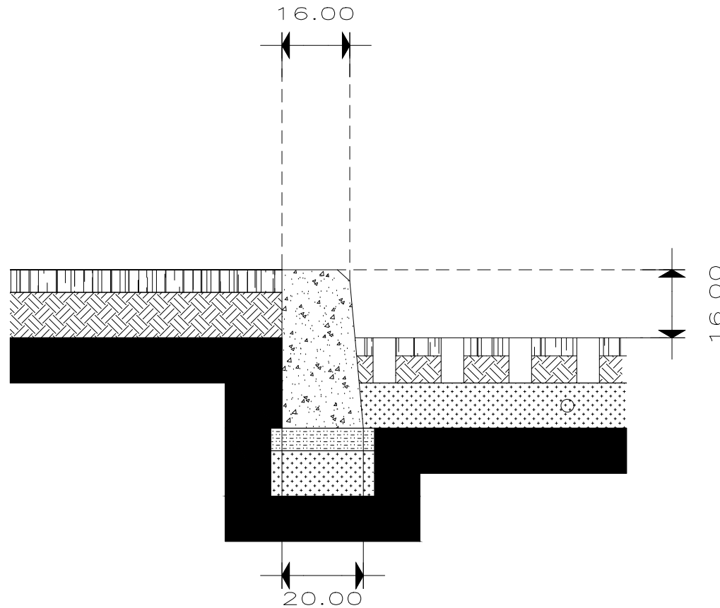
SECCIÓN GUARNICIÓN
